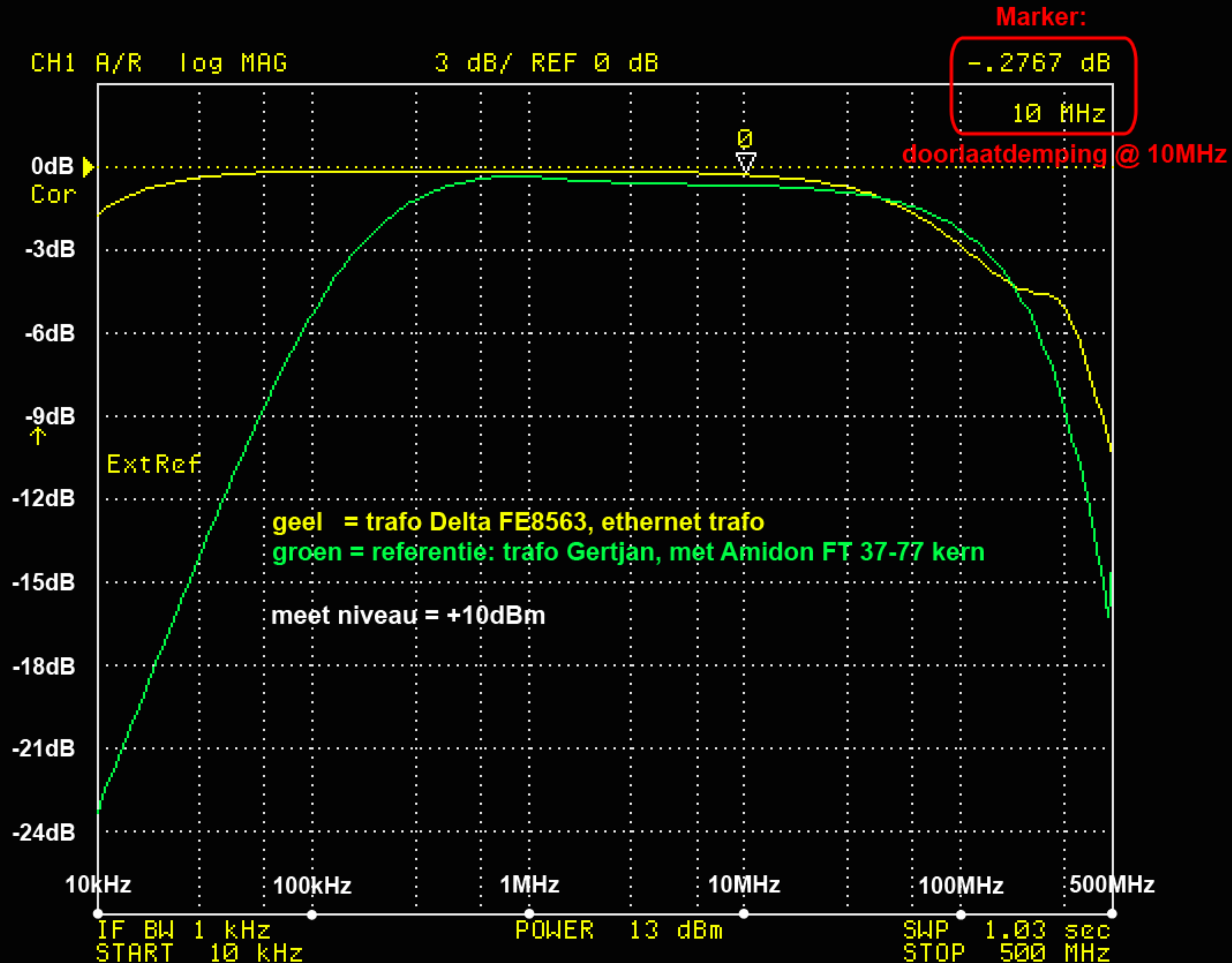
10MHz trafo "Delta FE8563", ethernet trafo frequentiecurve en doorlaatdemping
