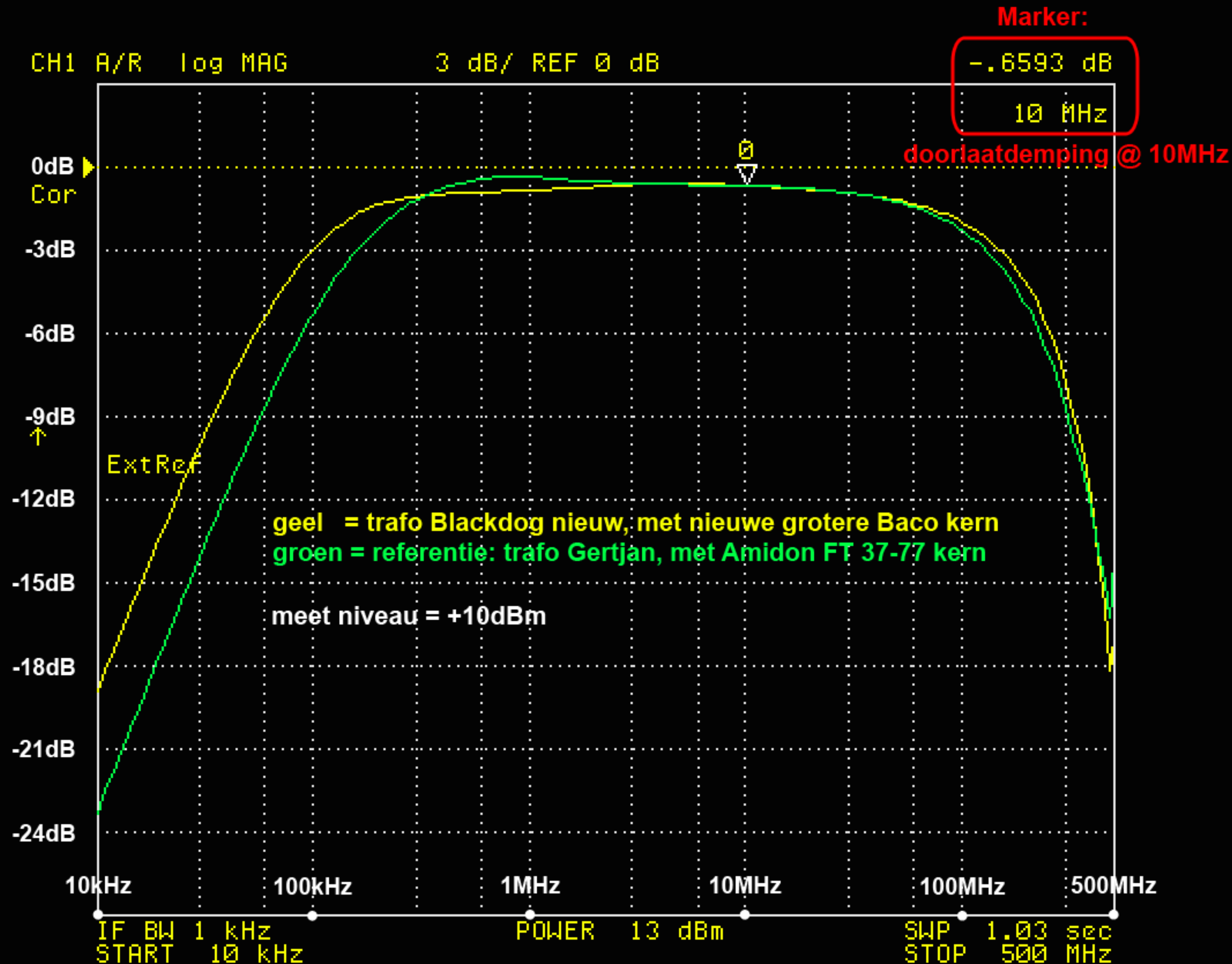
10MHz trafo "Blackdog nieuw", met nieuwe grotere Baco kern frequentiecurve en doorlaatdemping
