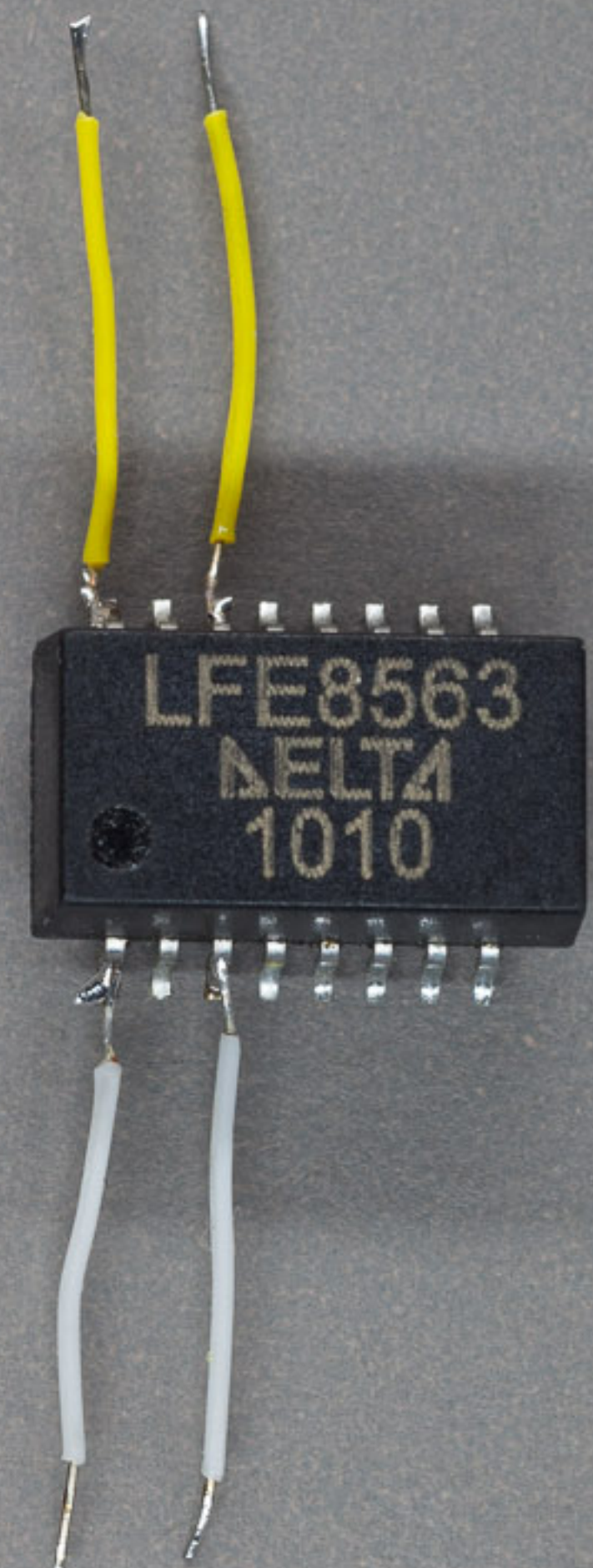
ethernet trafo
