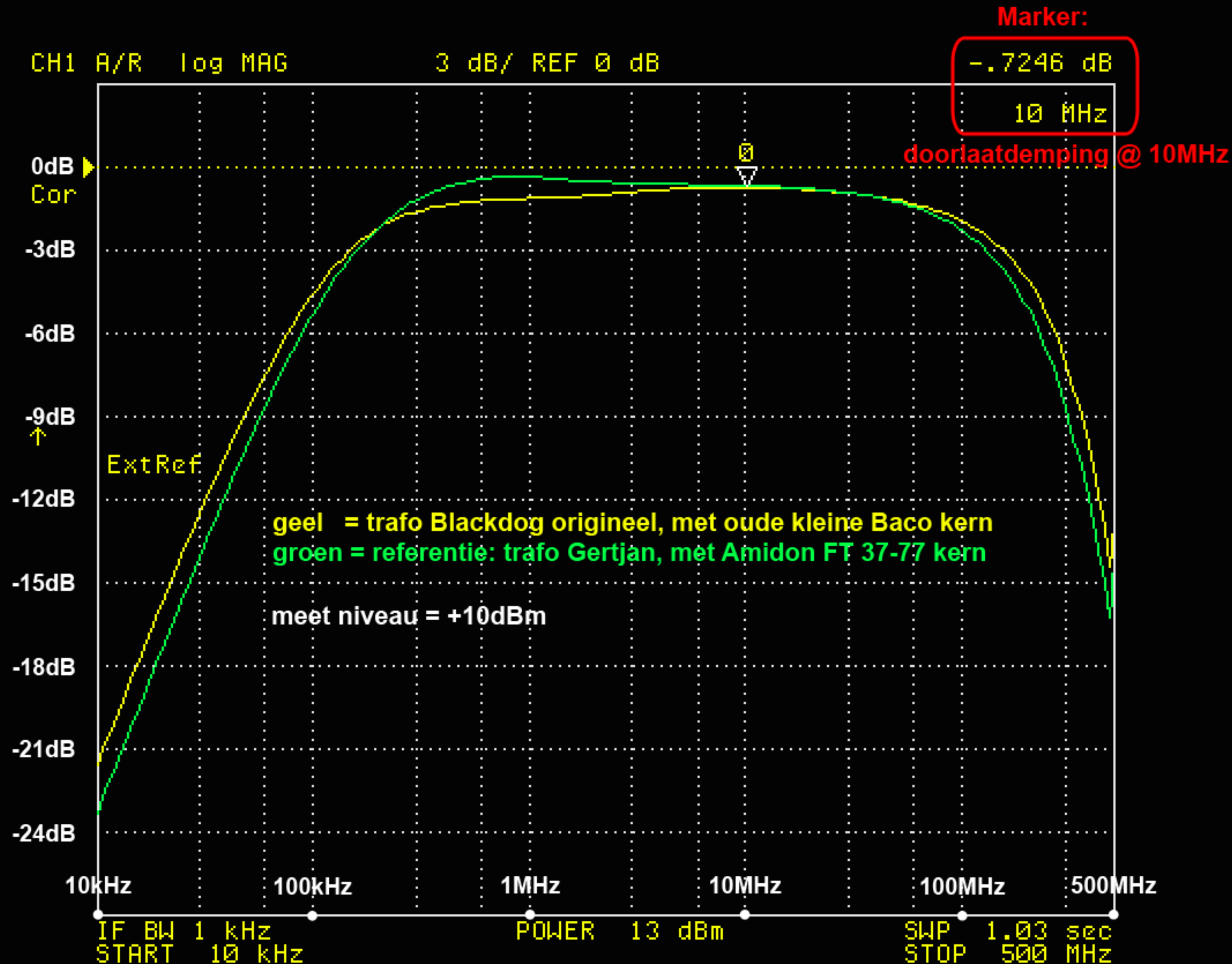
10MHz trafo "Blackdog origineel", met oude kleine Baco kern frequentiecurve en doorlaatdemping
