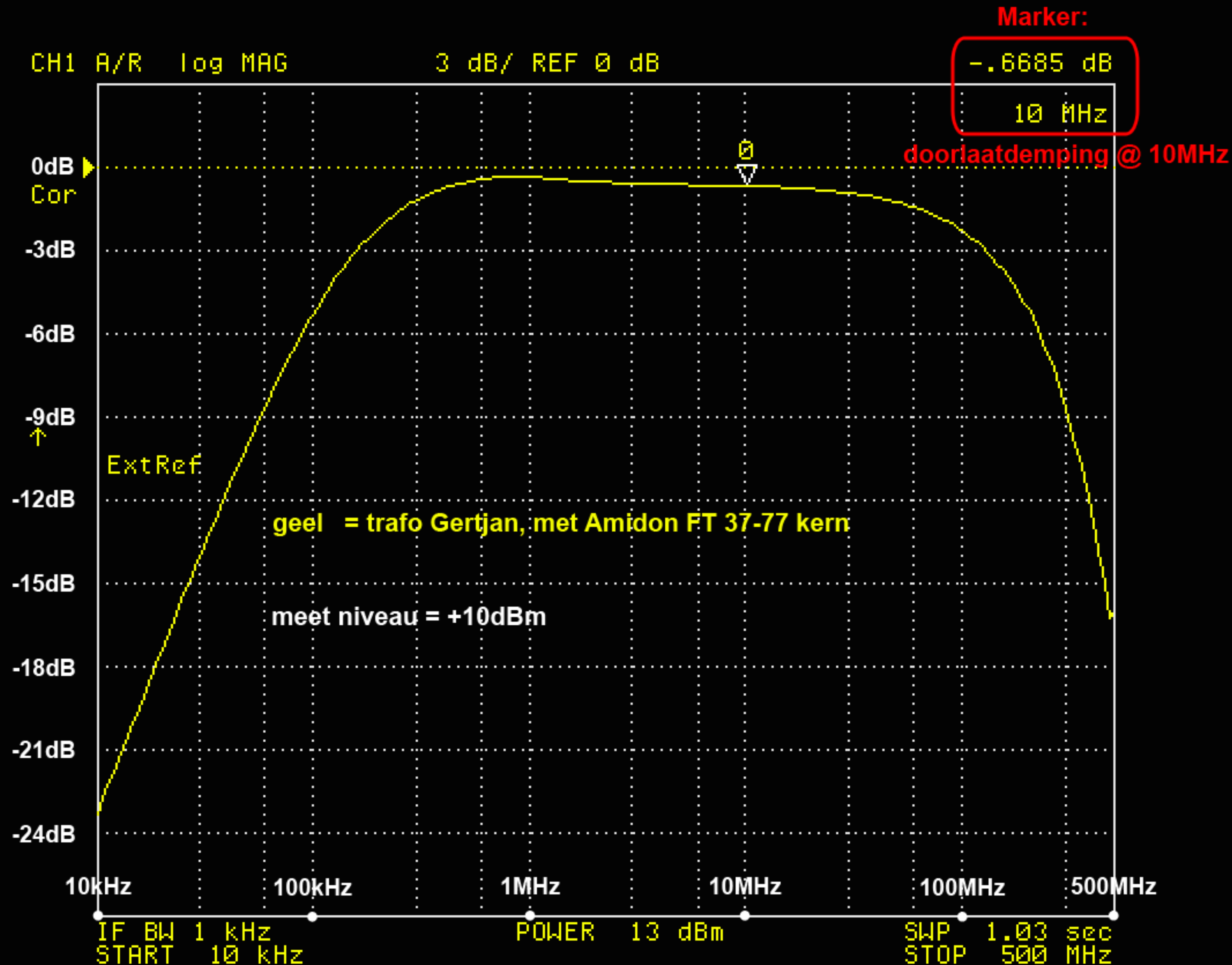
10MHz trafo “Gertjan”, met Amidon FT 37-77 kern frequentiecurve en doorlaatdemping
