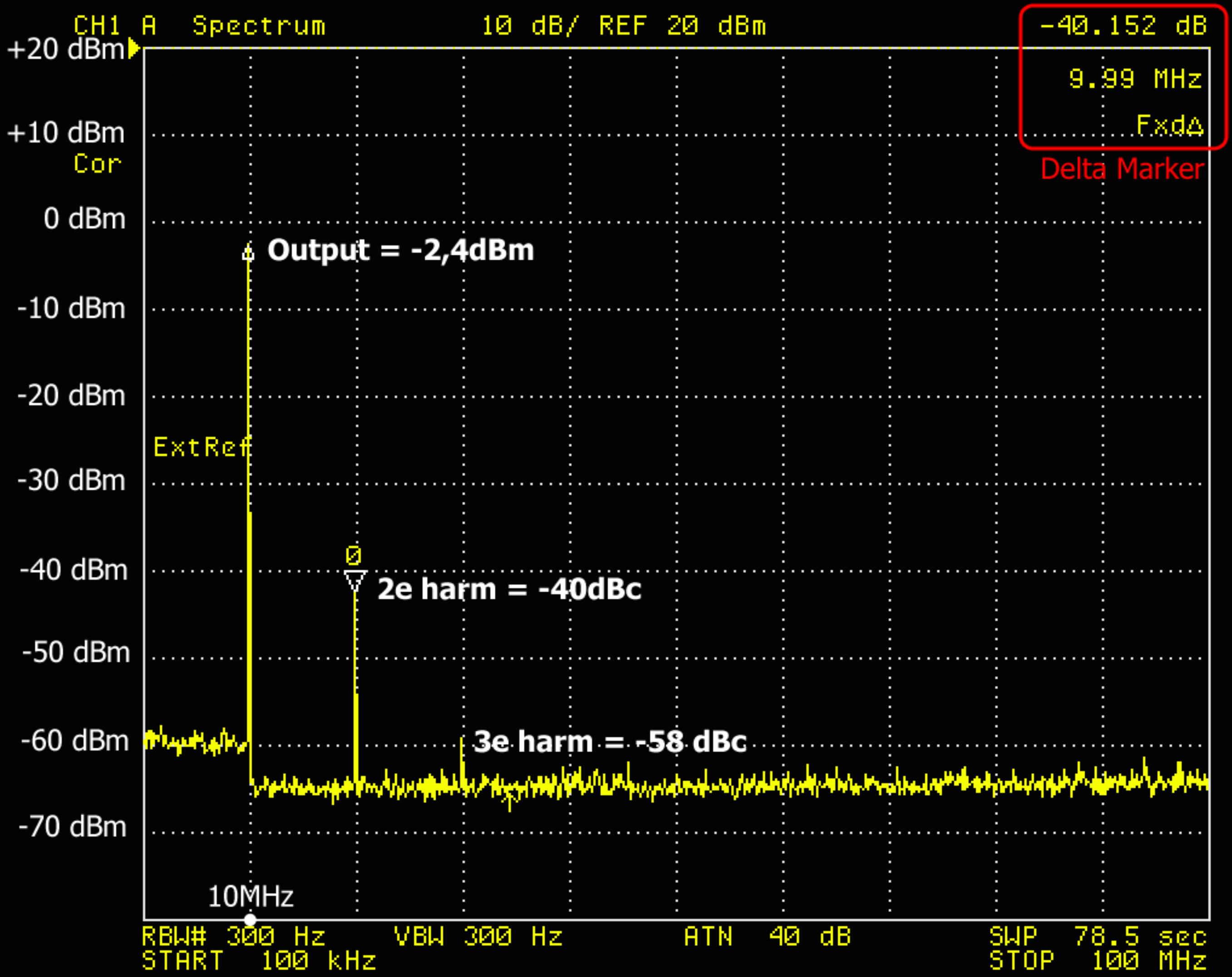
OCXO Oscilloquartz 8666-X nr.9543 output & harmonischen
