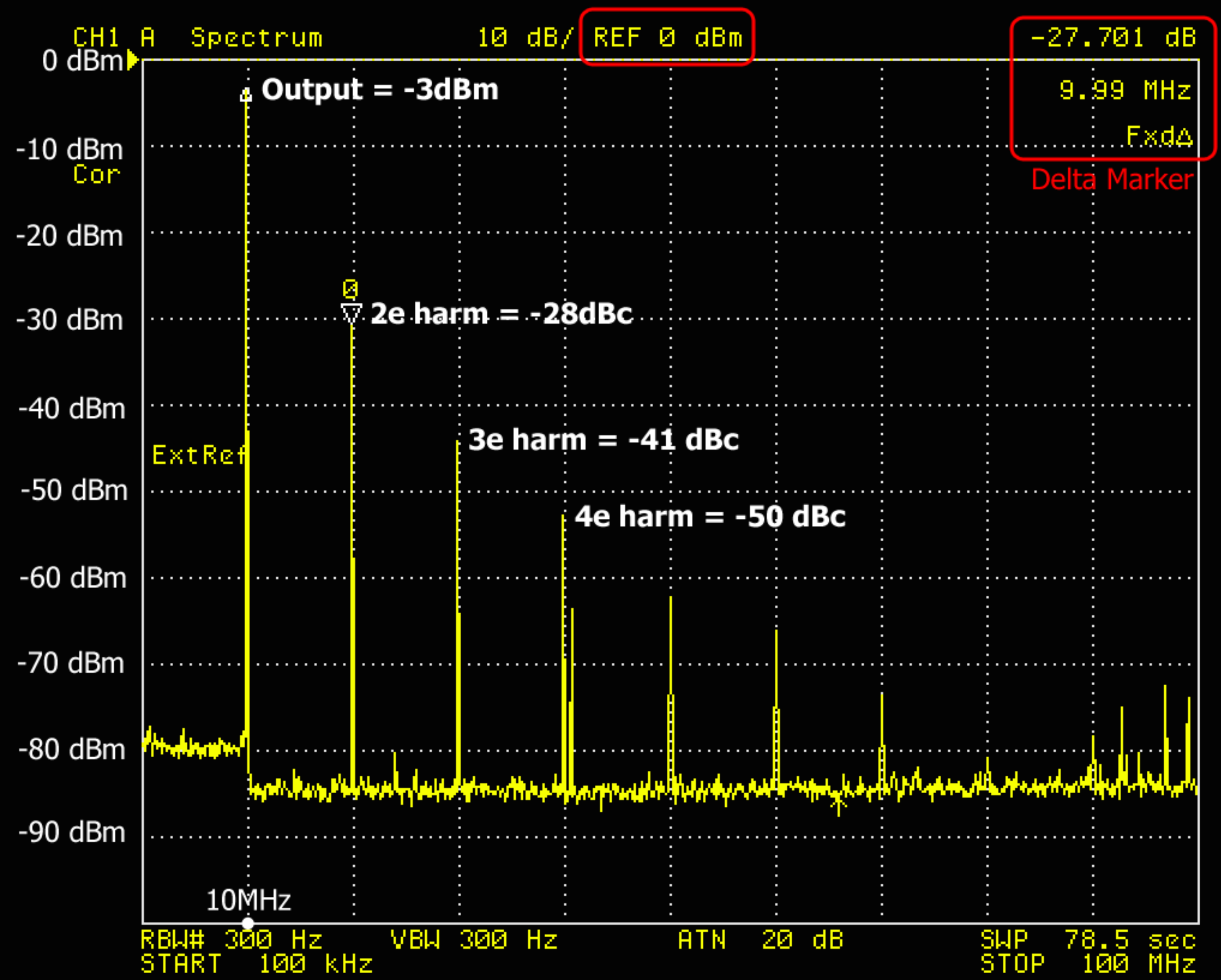
OCXO Oscilloquartz 8660-A nr.1828 output & harmonischen
