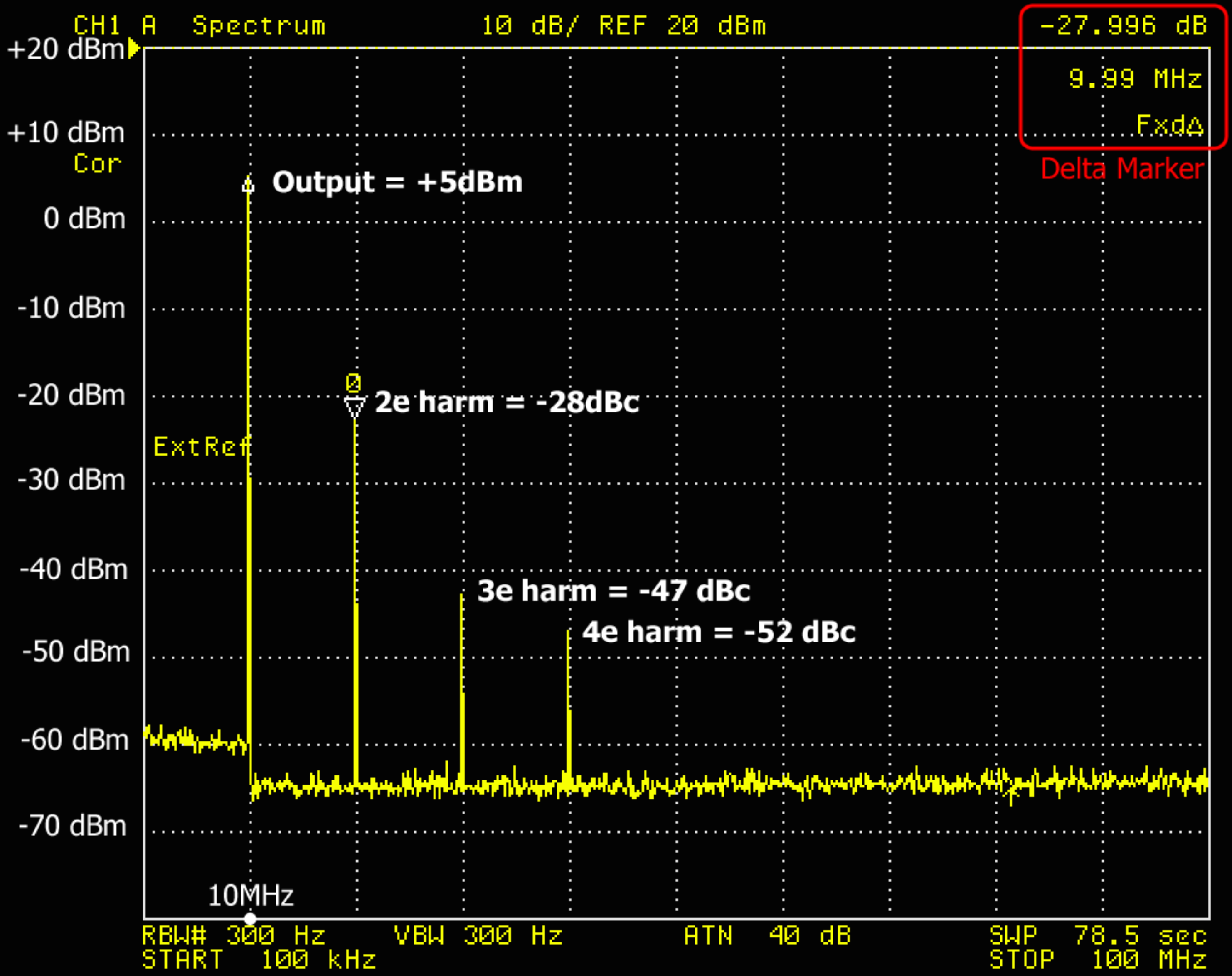
OCXO UCT 108663-02 nr. 5410 output & harmonischen
