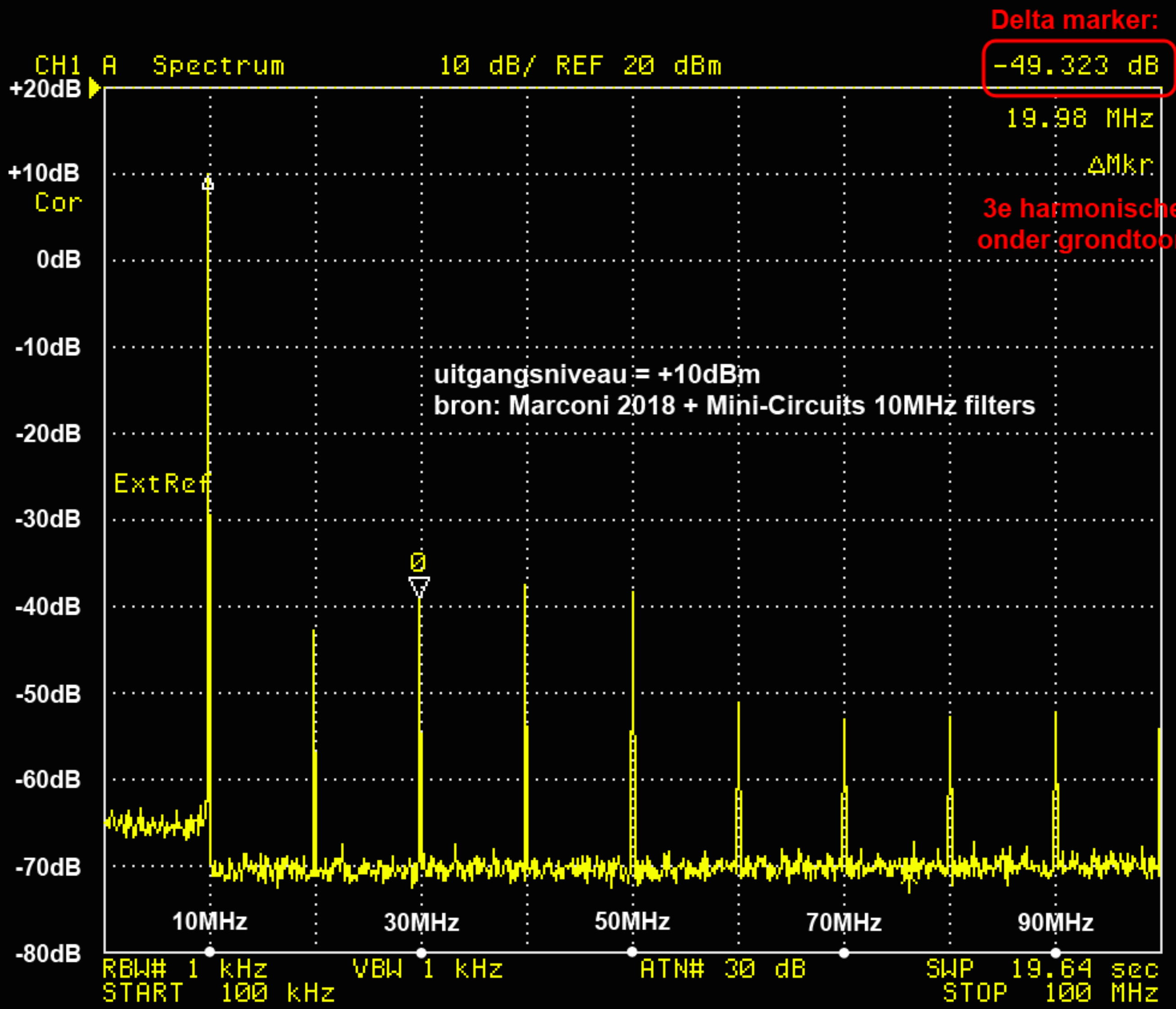
10MHz LM7171 uitgangstrap Masterclock - spectrum voeding: 12V, configuratie: standaard
