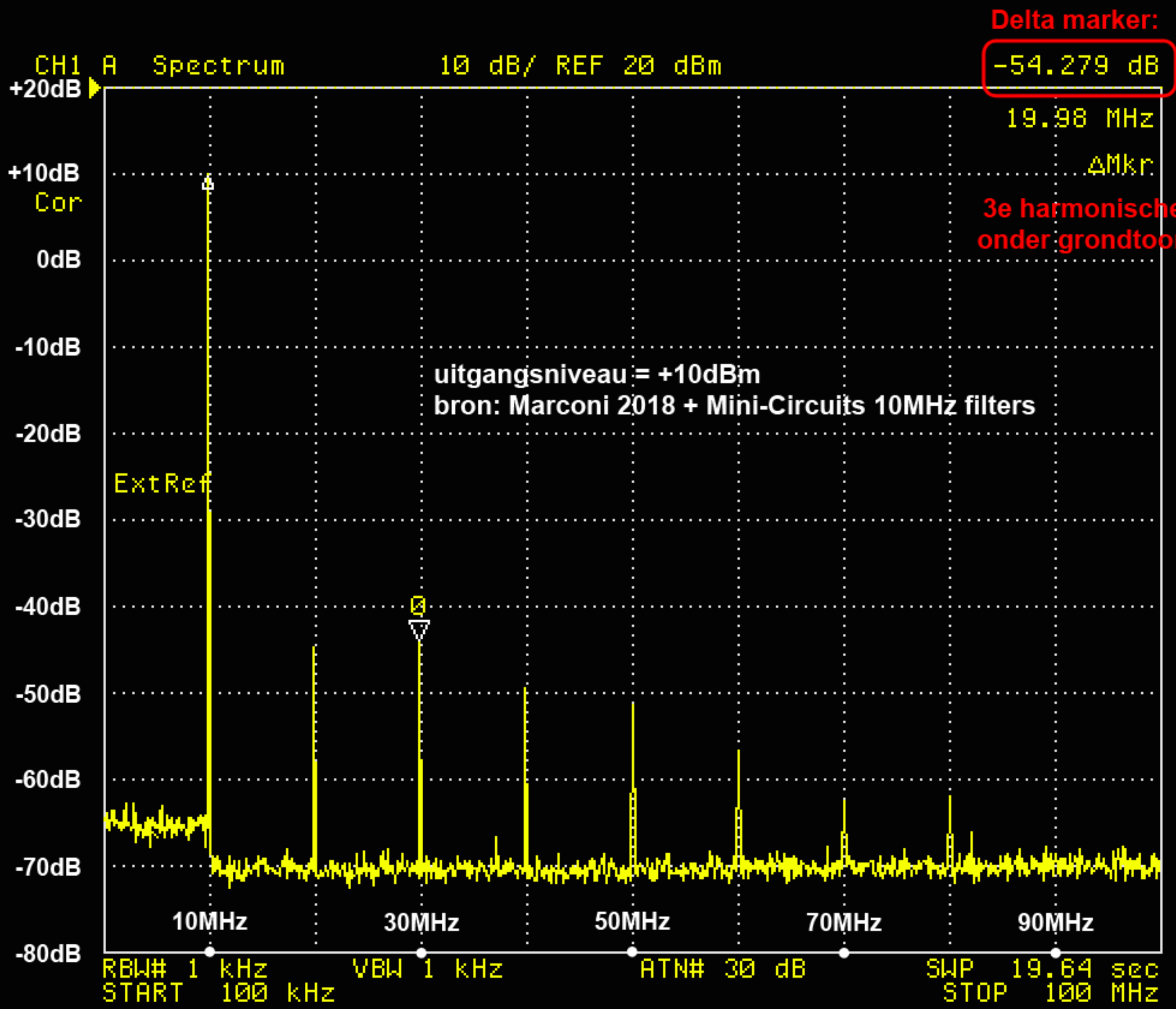
10MHz LM7171 uitgangstrap Masterclock - spectrum voeding: 24V, configuratie: standaard
