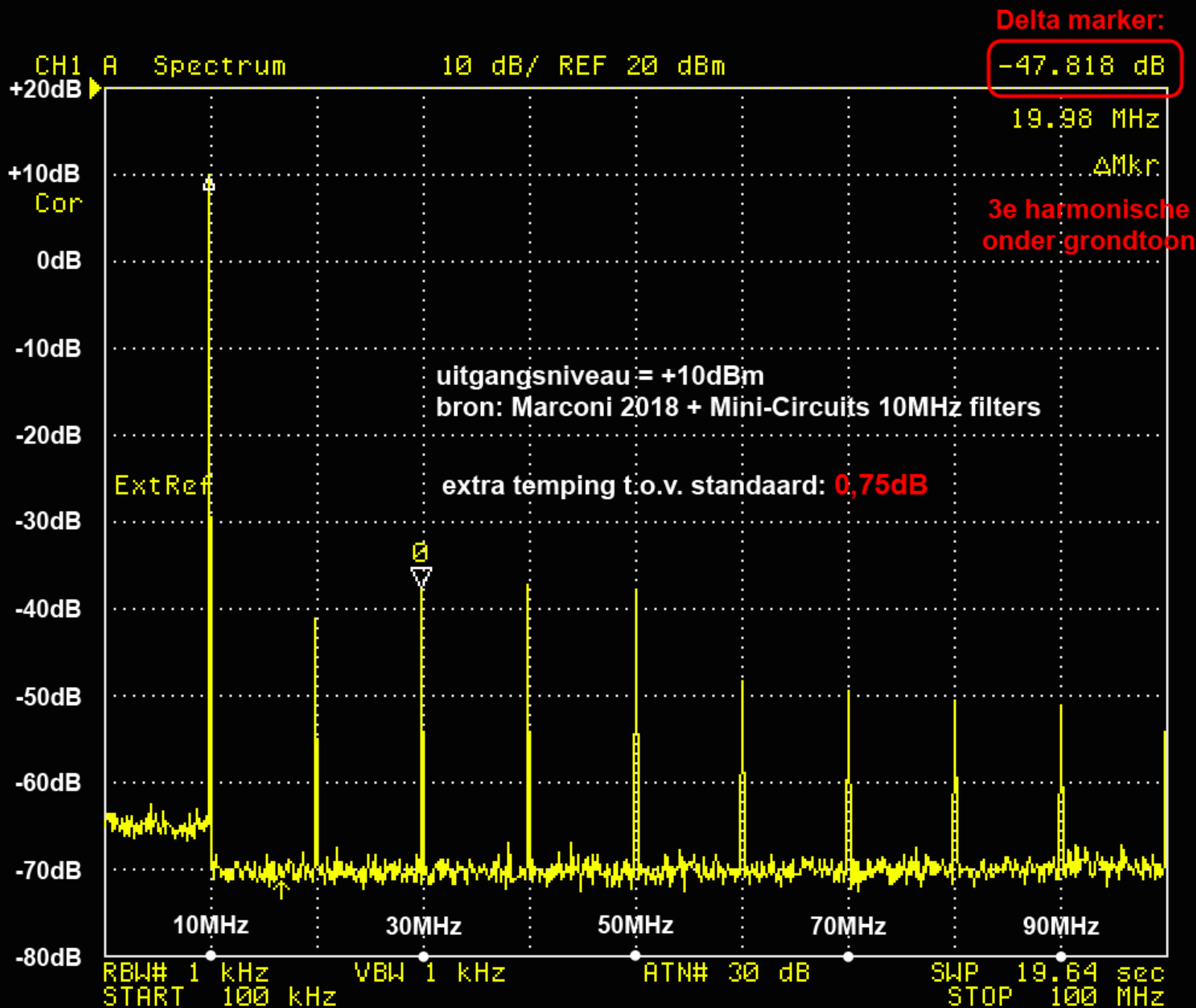
10MHz LM7171 uitgangstrap Masterclock - spectrum
