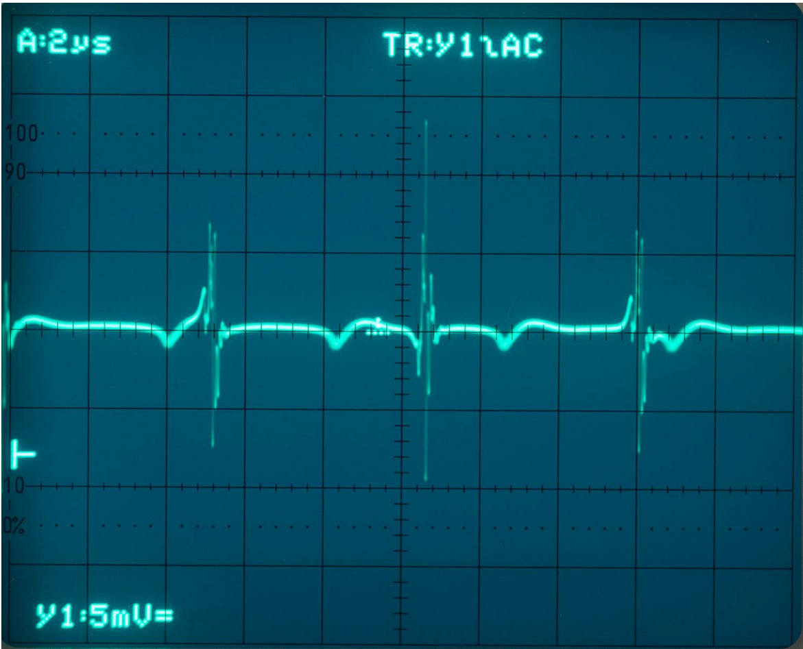
XP power DC-DC - strooiveld (probe lus)
