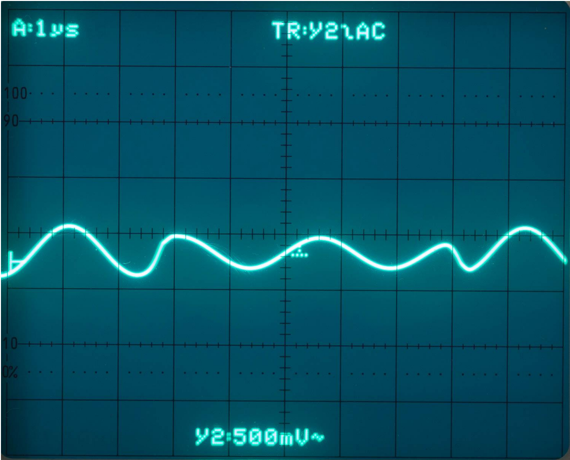
XP power DC-DC - strooiveld (oppikspoel)
