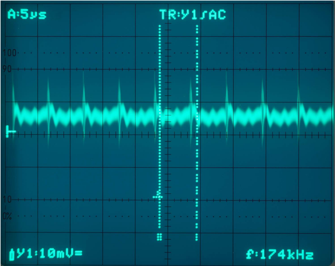
XP power DC-DC - lin (over 0,1R), zonder filters.
