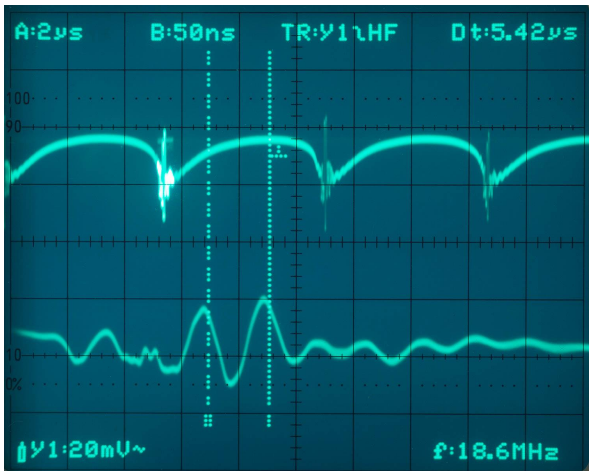
XP power DC-DC - Uuit zonder filters (load 2x50mA, piek uitvergroet, met markers
