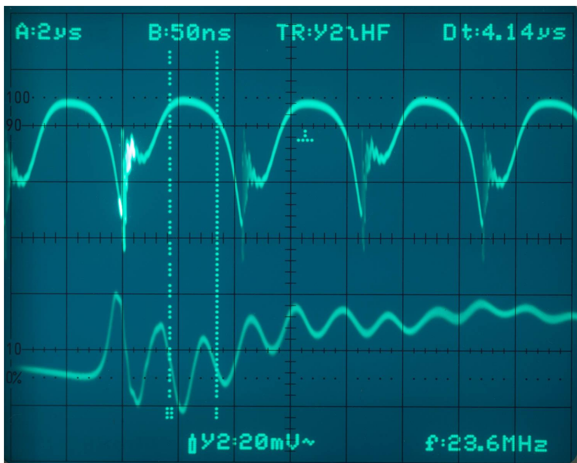
muRata DC-DC - Uuit zonder filters (load 2x50mA), piek uitvergroet, met markers
