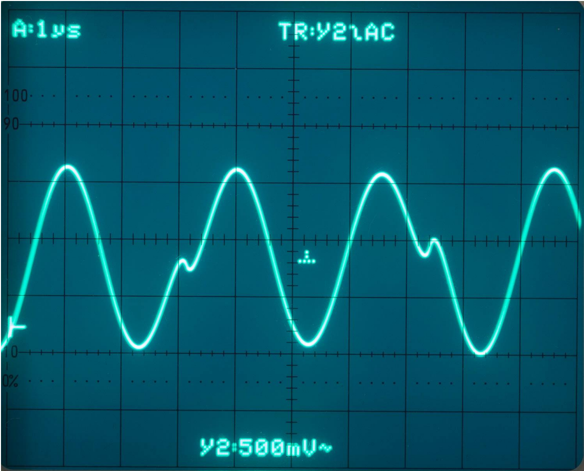
muRata DC-DC - strooiveld (oppikspoel)
