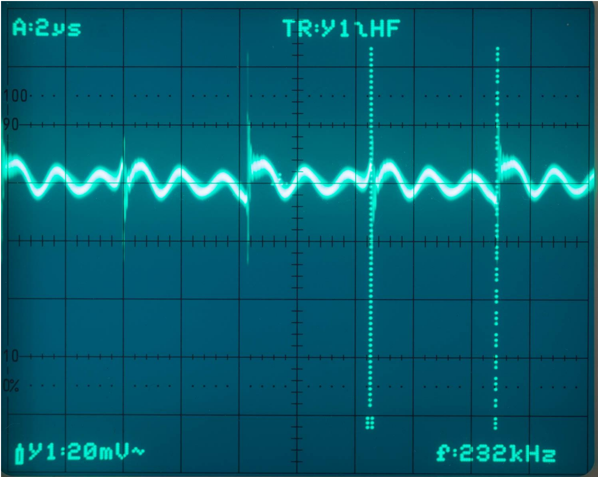
muRata DC-DC - lin (over 0,1R), zonder filters (load 2x50mA)
