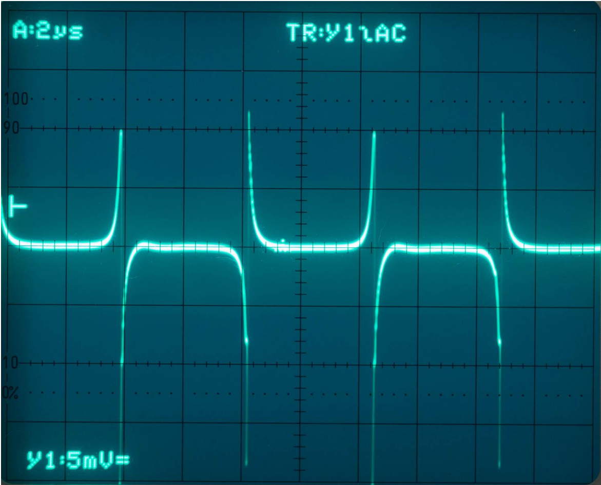
muRata DC-DC - strooiveld (probe lus)
