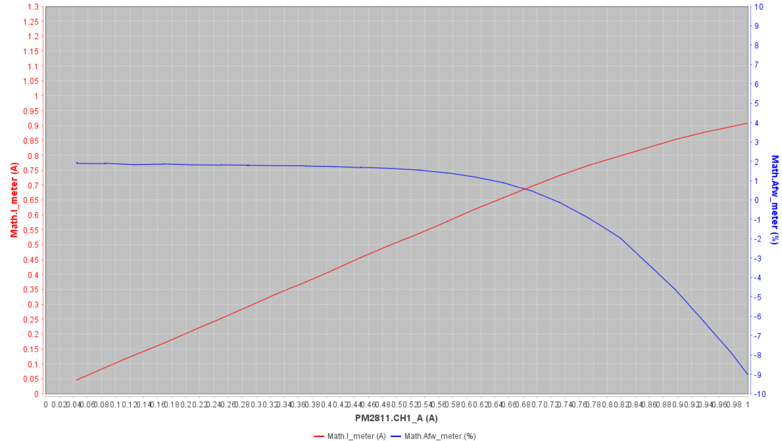
Stroommeter limiter - tot 1A
