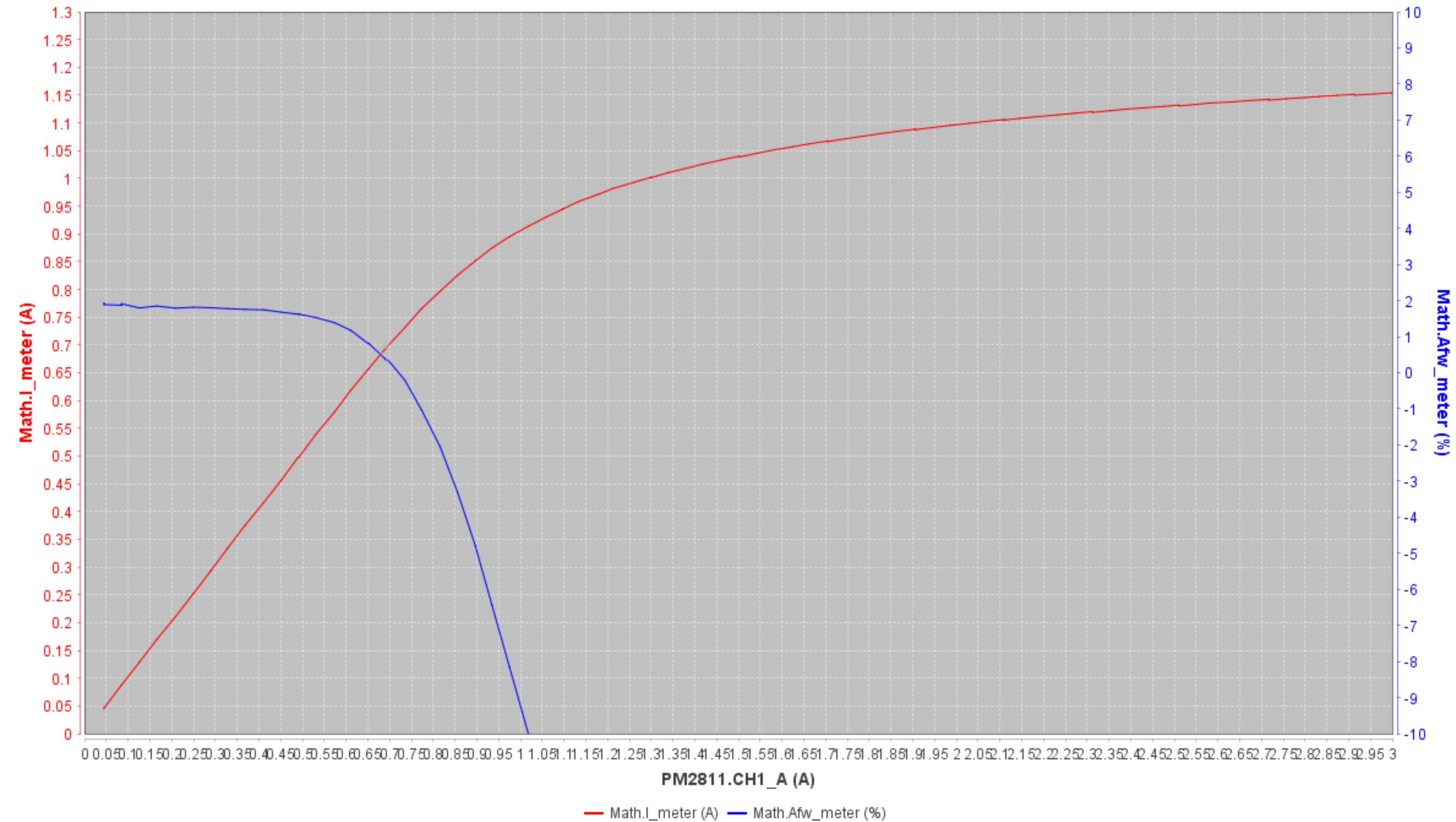
Stroommeter limiter - tot 3A
