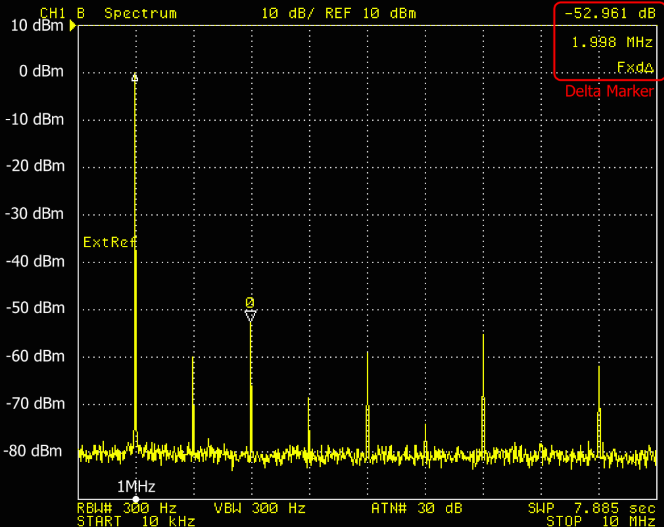
HP 8640B @ 1MHz / 0dBm out output & harmonischen
