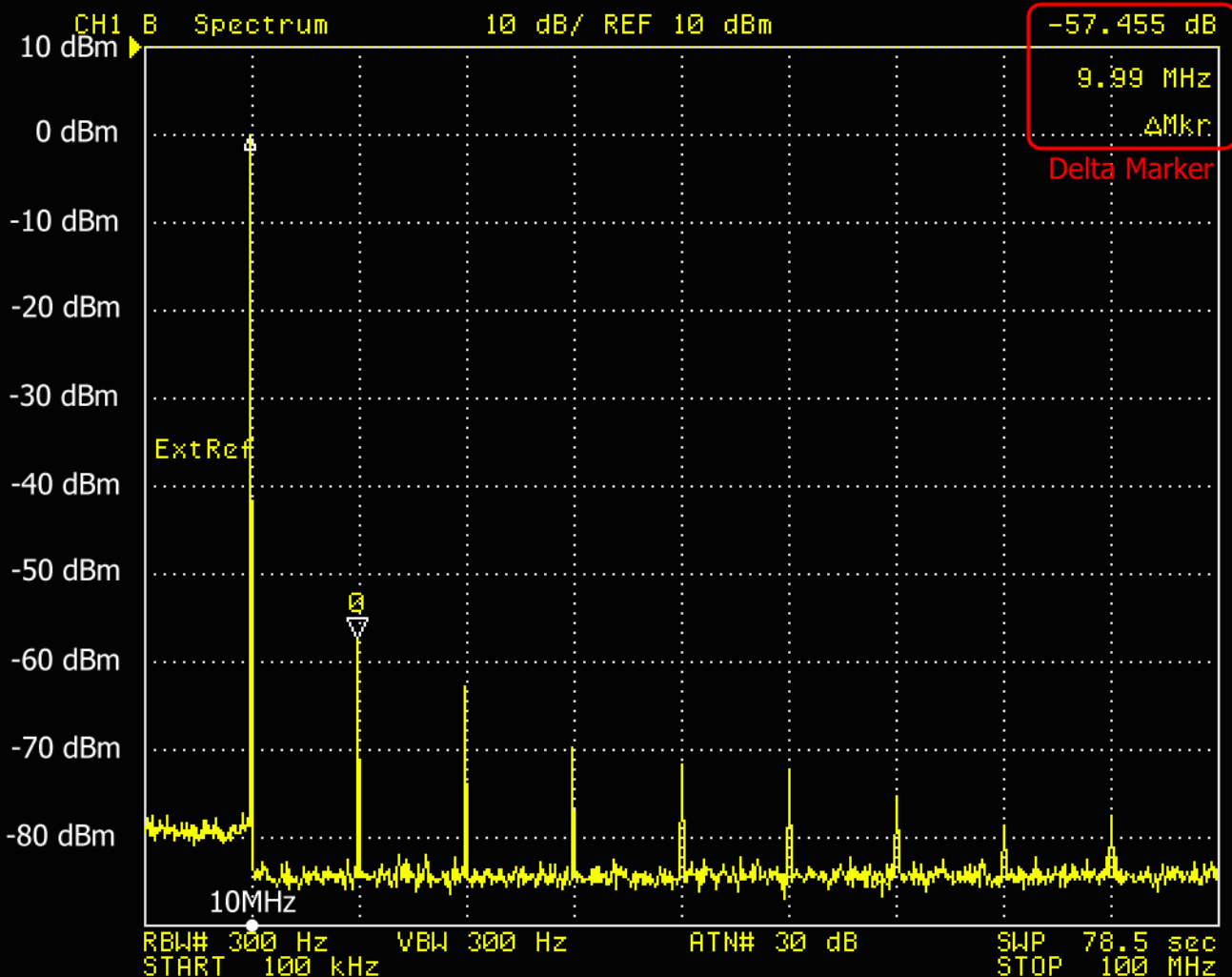
HP 8640B @ 10MHz / 0dBm out output & harmonischen
